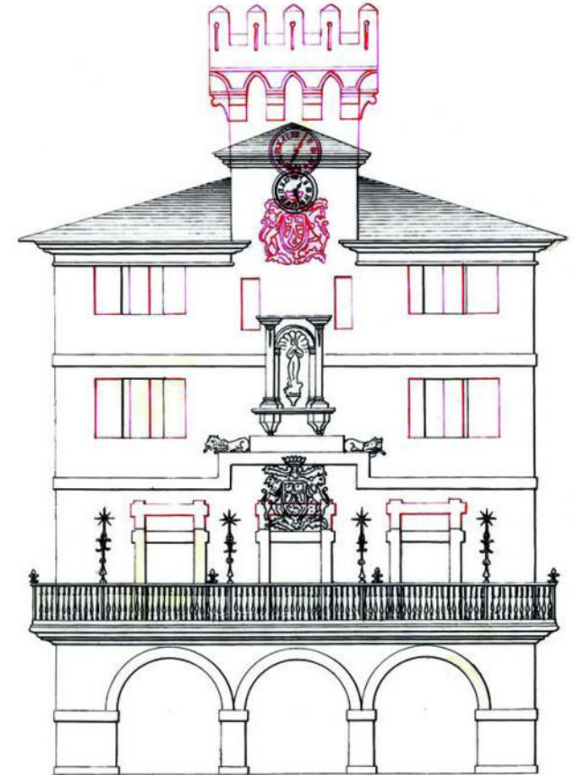
Plano de reforma de la Casa Consistorial de Eladio Laredo (1908)
