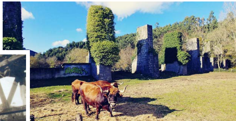
Pilastras de Dombergón en el valle de Sámamo. 10 pilares de sección trapezoidal construidos en silería y sillarejo caliza de planta cuadrada de 7 m. de lado y estructura trapezoidal, alcanzan 11,25 m. de altura. Sobre ellos se sostenían las vías del ferrocarril minero de Castro Alén que vadeaba en este punto la carretera de Hoz y el río de Sámamo. Fueron construidas hacia 1890.
